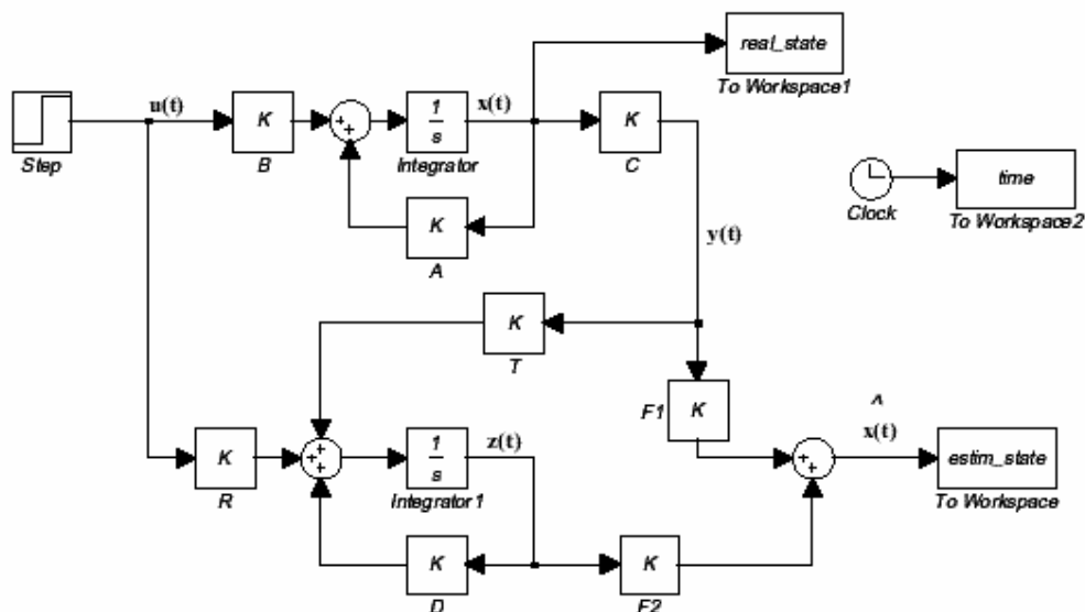
شکل ض ۱-۱-۱۰- فایل reduced_observer.mdl مورد استفاده در برنامه شکل ض ۱-۹
